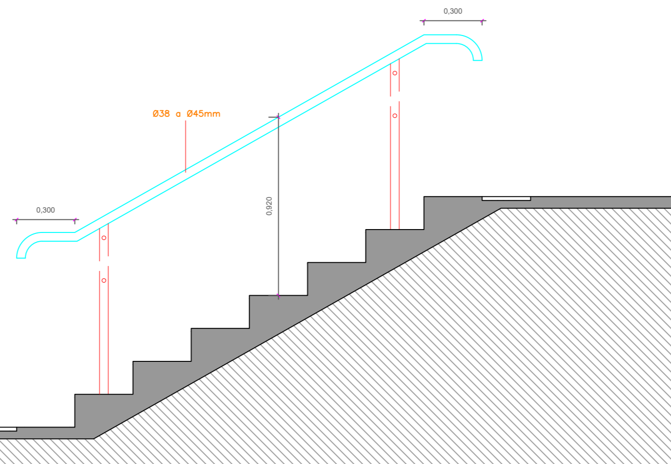
DET. 04 - CORRIMÃO DAS ESCADAS
