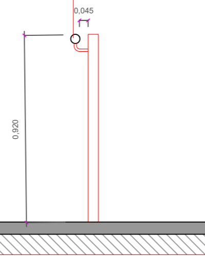
VISTA FRONTAL CORRIMÃO DAS ESCADAS
