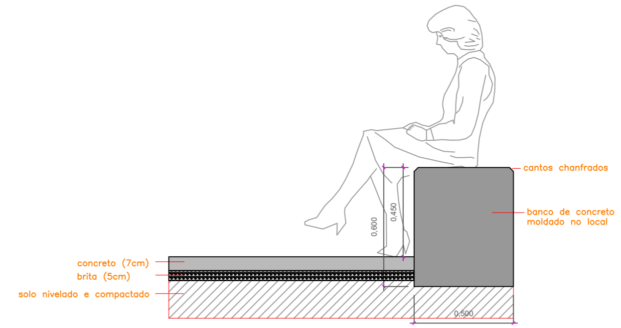
DET. 06 - BANCO DE CONCRETO X PISO CONCRETO
