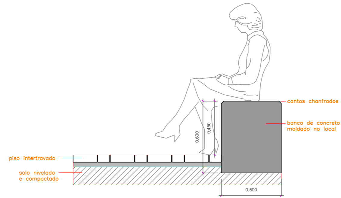
DET. 05 - BANCO DE CONCRETO X INTERTRAVADO
